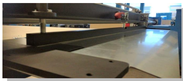
Handschere mit Niederhalter (gummiert) und Obermesser mit integrierter Führungsrolle
