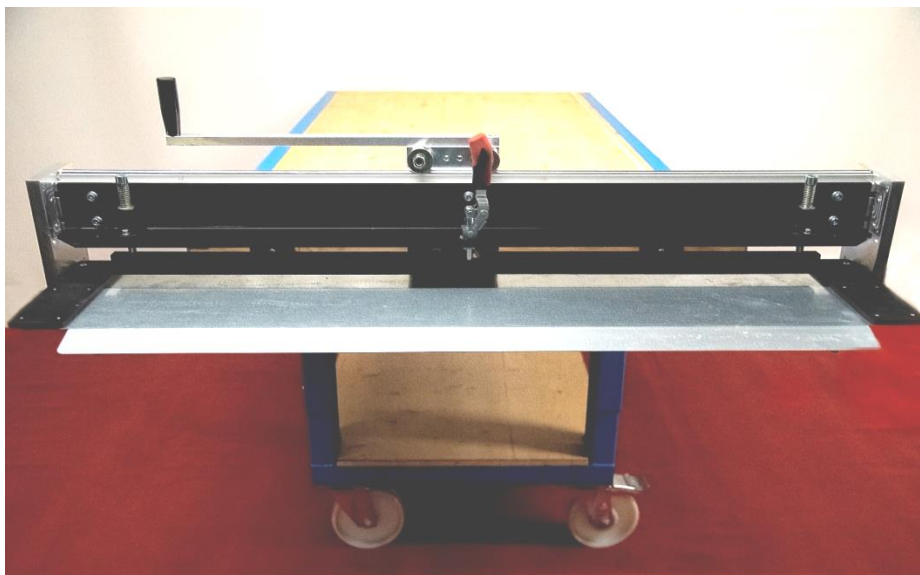
Zuschneid- und Ablängtisch optional mit Handschere TS1000 oder TS1250mm
